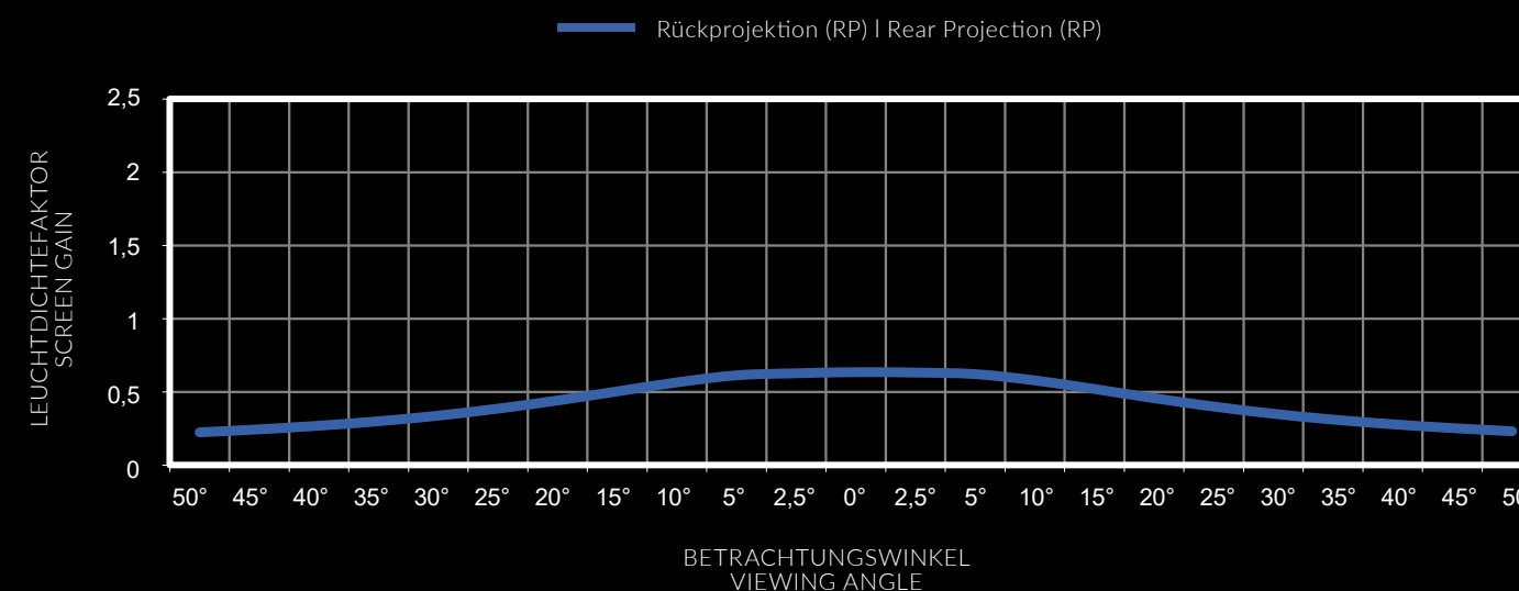
LEUCHTDICHTEFAKTOR NACH DIN 19045 | GAIN ACCORDING TO DIN 19045 FLEX REAR PRO
