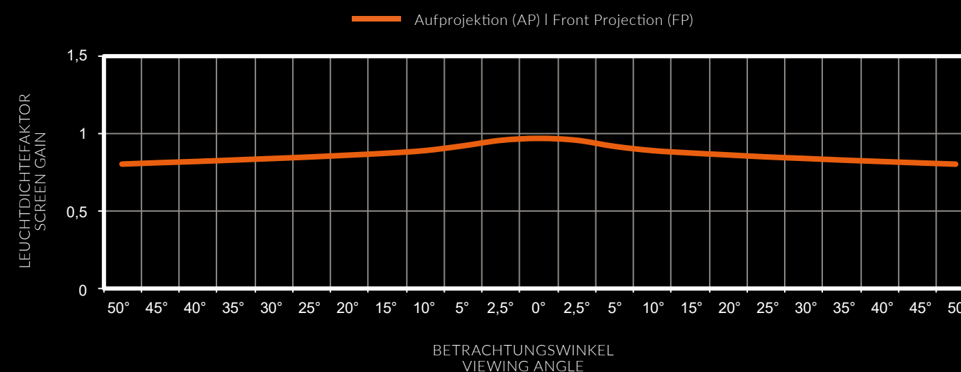
LEUCHTDICHTEFAKTOR NACH DIN 19045 | GAIN ACCORDING TO DIN 19045 FLEX WHITE OPAQUE
