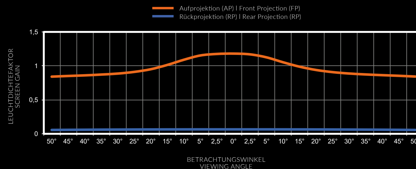
LEUCHTDICHTEFAKTOR NACH DIN 19045 | GAIN ACCORDING TO DIN 19045 FLEX WHITE MO
