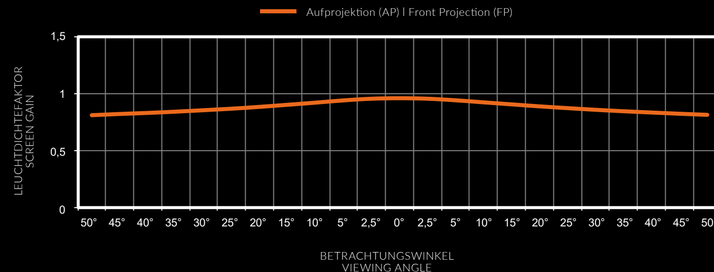
LEUCHTDICHTEFAKTOR NACH DIN 19045 | GAIN ACCORDING TO DIN 19045 FLEX WHITE BLACK CI
